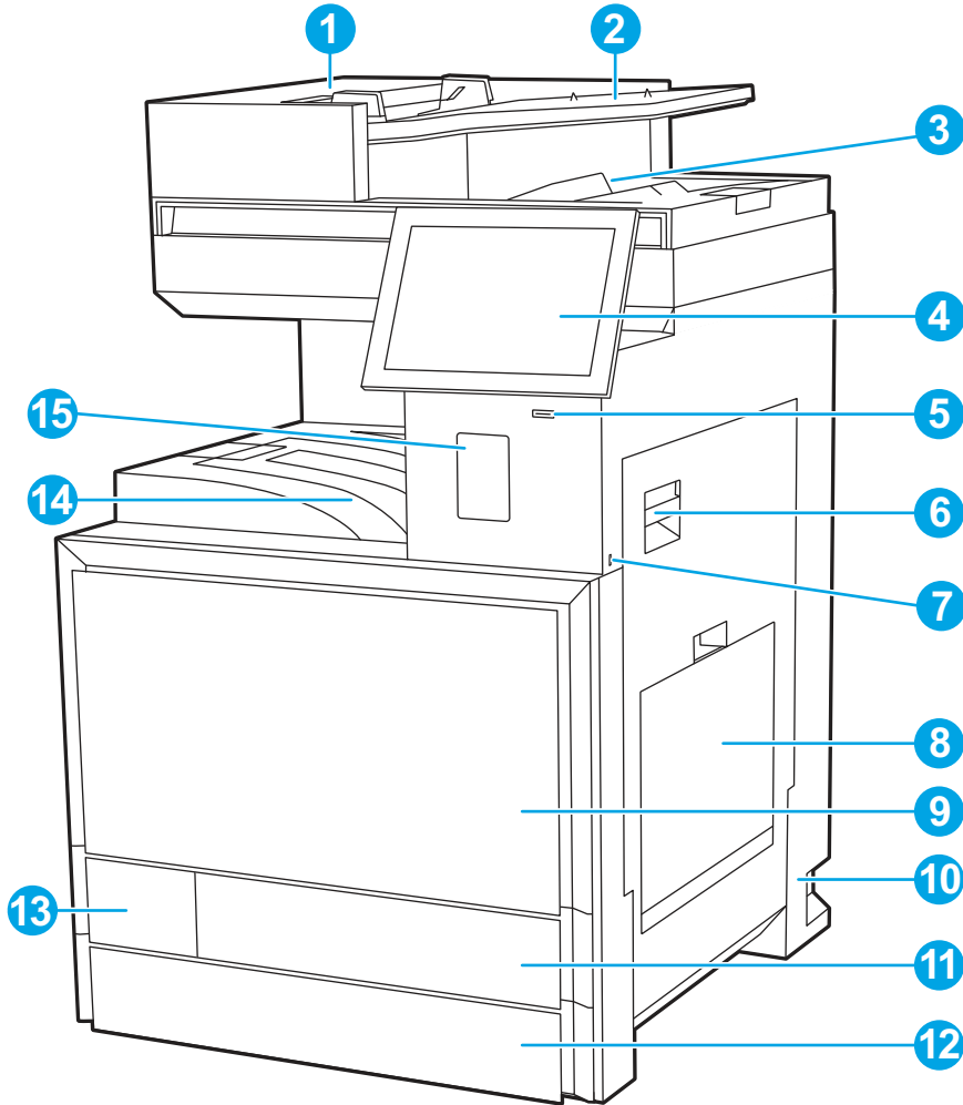
Figura 1-6 Vista frontal da impressora
