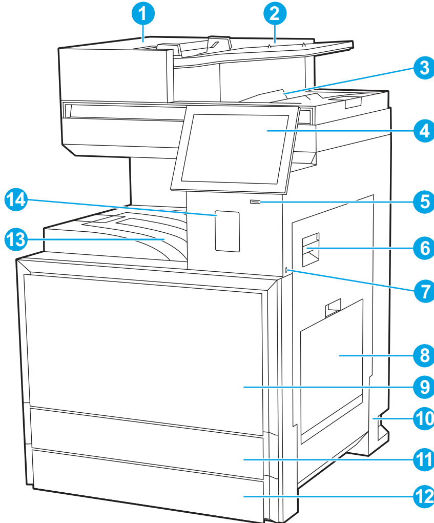
Figura 1-6 Vista frontal da impressora
